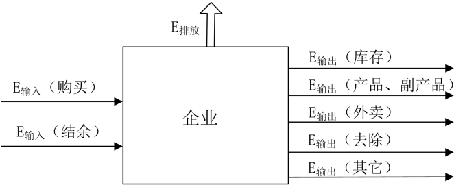
图 G.1 黑箱物料平衡法原理示意图
