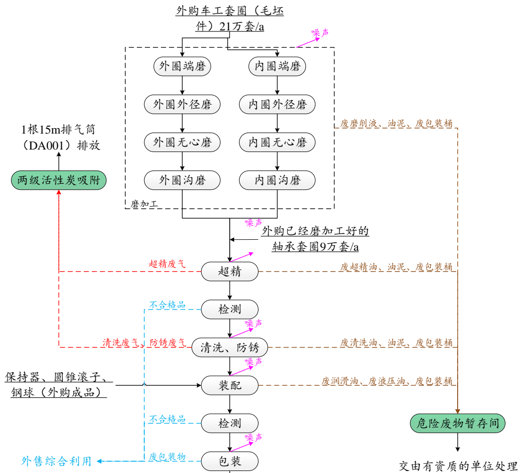
图2 一期工程轴承生产工艺流程及产污节点图
