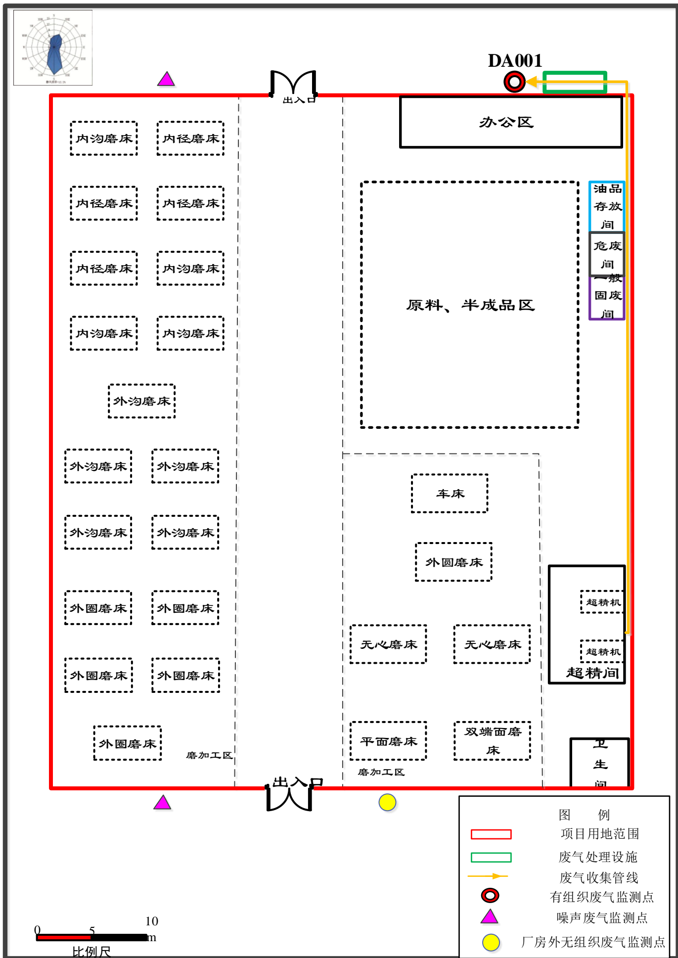
附图3 厂区平面布置图(1F)
