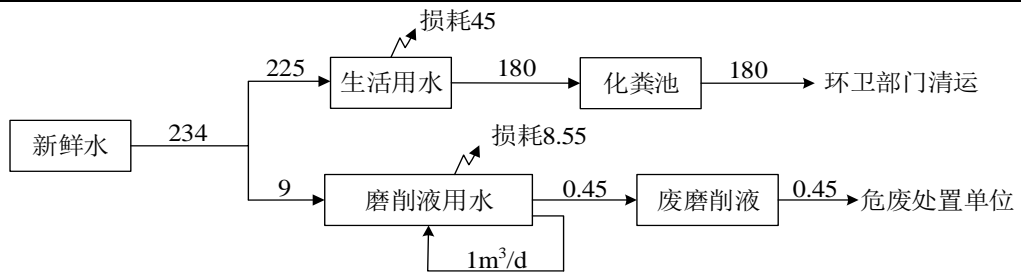
图1 项目一期工程水平衡图（单位： m^3/a ）
