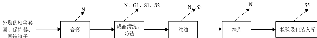
图2 一期工程轴承生产工艺流程及产污节点图
